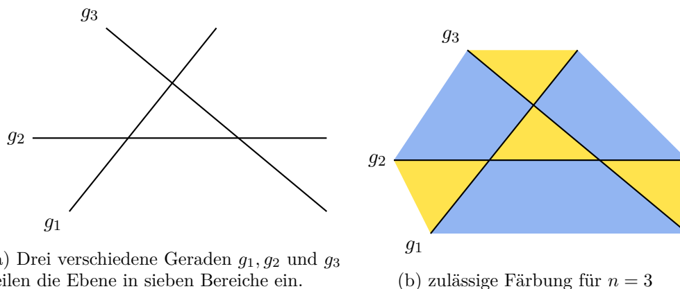
Abbildung 2.4: zulässige Färbung für drei Geraden
