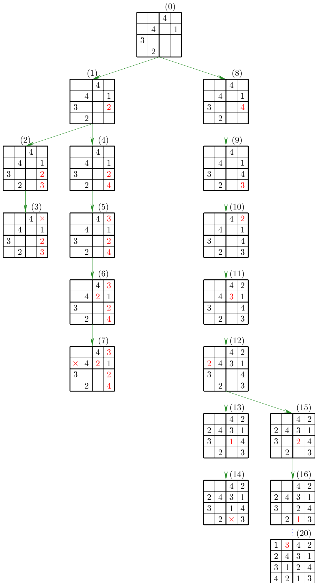
Abbildung 6.8: Visualisierung von Backtracking bei Sudoku
